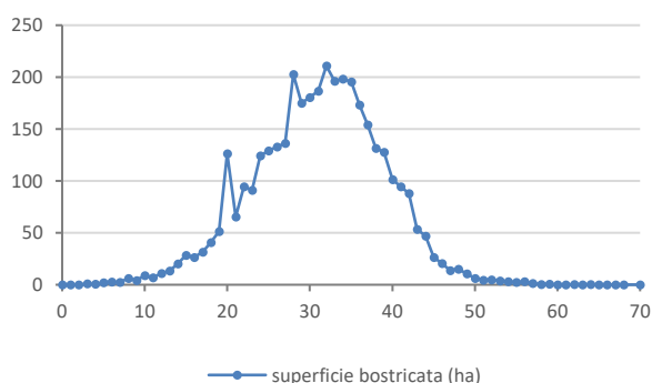
Correlazione tra la pendenza media (espressa in gradi) in ognuna delle aree infettate e la loro estensione (in ha). La curva mostra che la metà delle aree individuate ha una pendenza media compresa tra i 28 e i 37 gradi.
