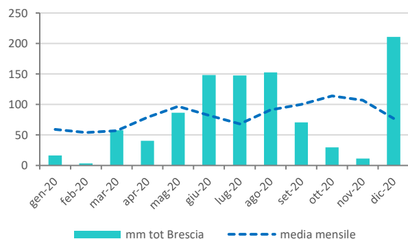
Andamento delle precipitazioni (mm pioggia cumulati su base mensile) in una stazione di rilevamento mediamente a piovosità ordinaria (Brescia), rispetto alla media mensile del periodo 1990-2019.
