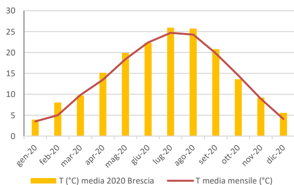
Andamento delle temperature medie mensili (°C) in una stazione di rilevamento dell'alta pianura (Brescia), rispetto alla media mensile del periodo 1990-2019.
