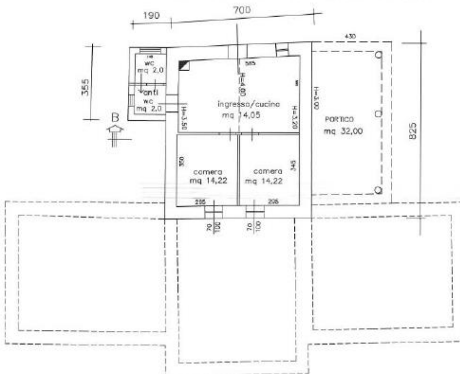
FABBRICATO CAMPOLUNGO INFERIORE PIANO RIALZATO Scala 1:100
