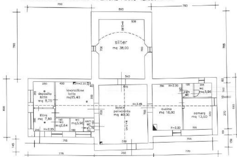
FABBRICATO CAMPOLUNGO INFERIORE PIANO TERRA Scala 1:100
